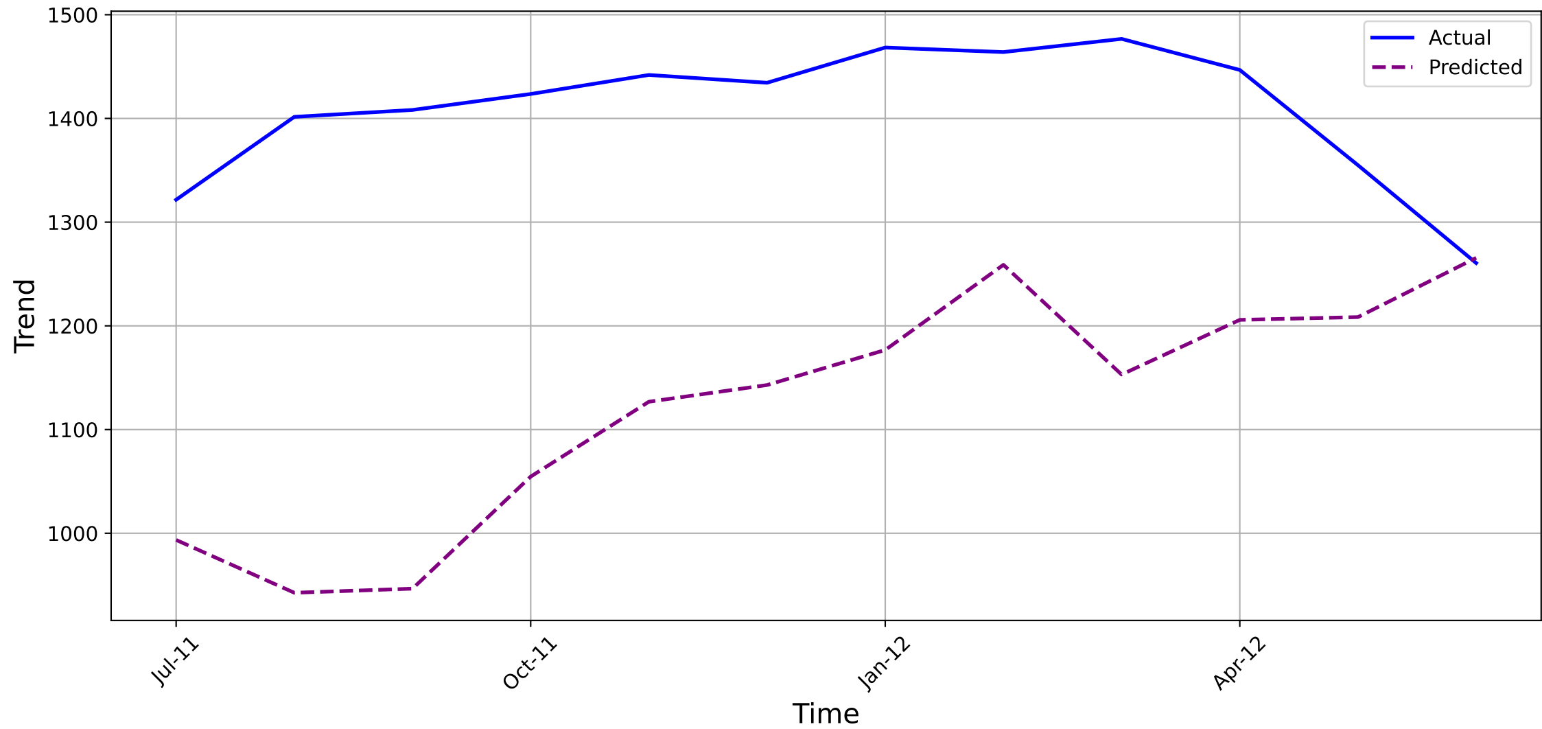
Malware-ALL - Validation
